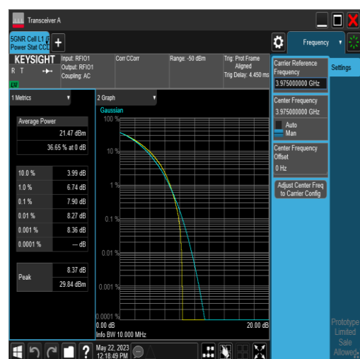
NTNV_N77-3700-3980_PC2_30_10_H_TID6_#1
