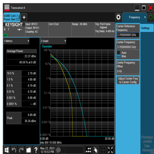
NTNV_N77-3700-3980_PC2_30_10_L_TID2_#1
