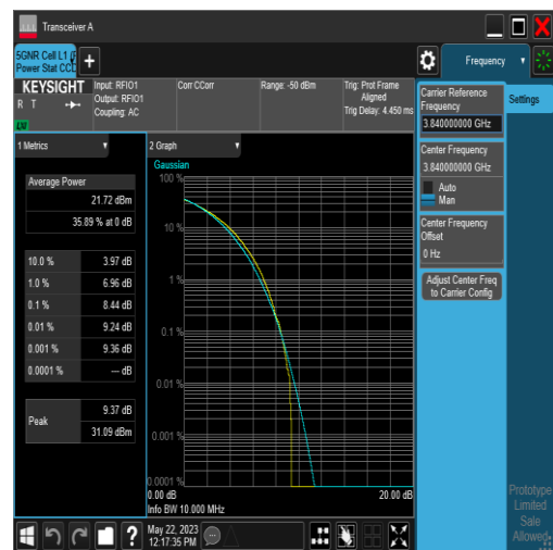
NTNV_N77-3700-3980_PC2_30_10_M_TID6_#1
