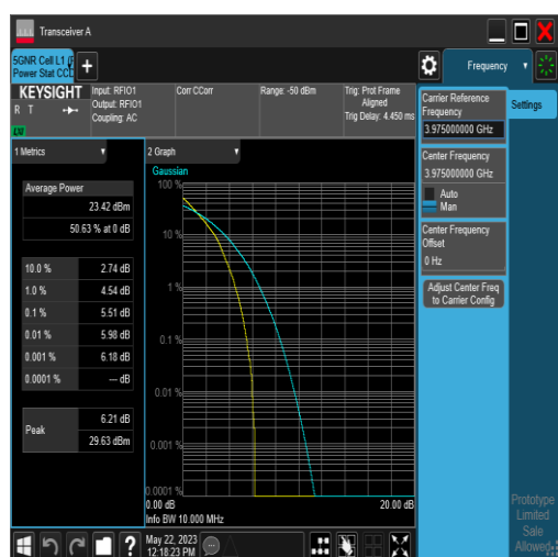
NTNV_N77-3700-3980_PC2_30_10_H_TID2_#1
