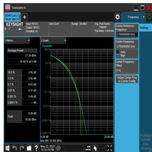
NTNV_N77-3700-3980_PC2_30_10_L_TID6_#1
