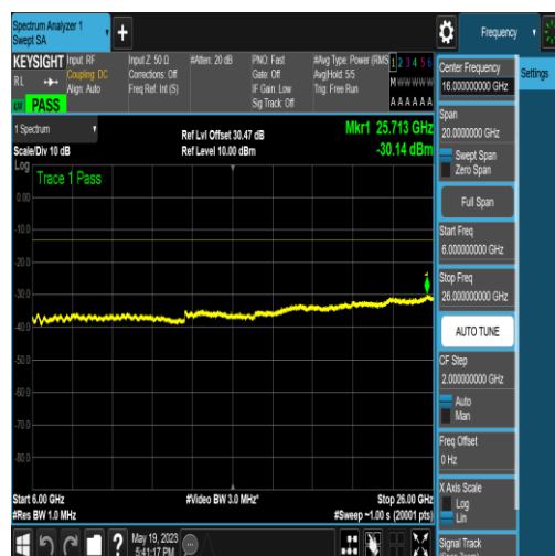
NTNV_N77-3700-3980_PC2_30_60_L_TID6_NS_ 01_6000_26000_#1
