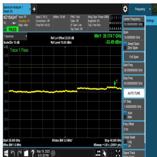
NTNV_N77-3700-3980_PC2_30_60_L_TID6_NS_ 01_26000_40000_#1
