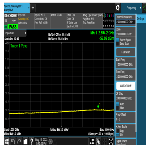
NTNV_N77-3700-3980_PC2_30_60_L_TID5_NS_ 01_1000_3000_#1
