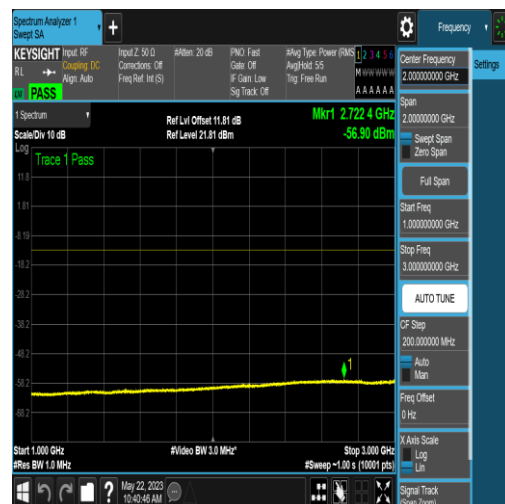
NTNV_N77-3700-3980_PC2_30_80_L_TID16_NS _01_1000_3000_#1
