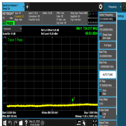
NTNV_N77-3700-3980_PC2_30_80_L_TID16_NS _01_30_1000_#1
