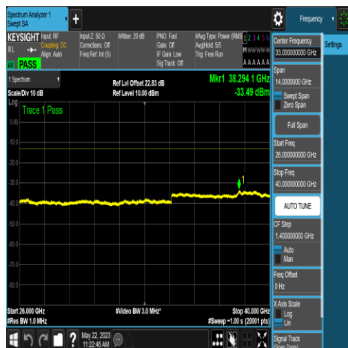
NTNV_N77-3700-3980_PC2_30_90_L_TID16_NS _01_26000_40000_#1
