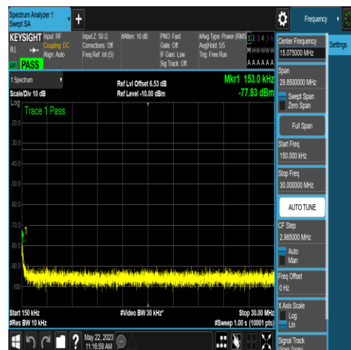
NTNV_N77-3700-3980_PC2_30_90_L_TID5_NS_ 01_0.15_30_#1
