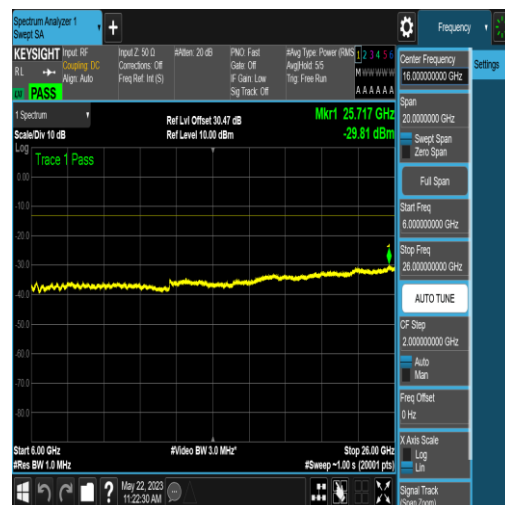
NTNV_N77-3700-3980_PC2_30_90_L_TID16_NS _01_6000_26000_#1
