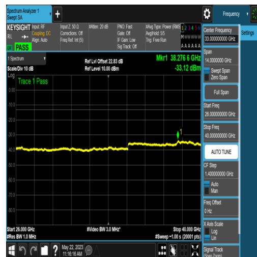
NTNV_N77-3700-3980_PC2_30_90_L_TID4_NS_ 01_26000_40000_#1
