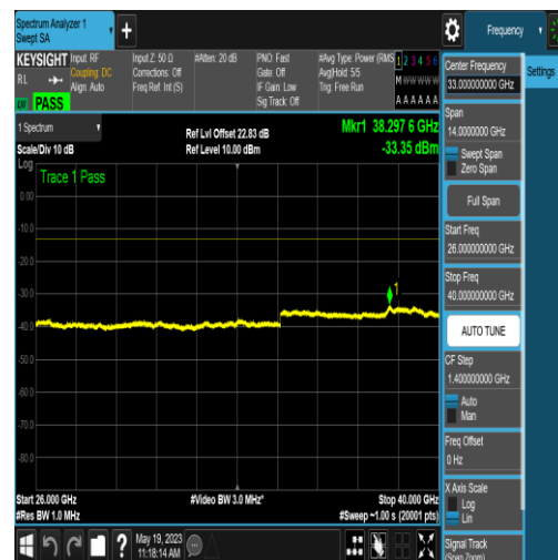
NTNV_N77-3700-3980_PC2_30_100_L_TID17_N S_01_26000_40000_#1
