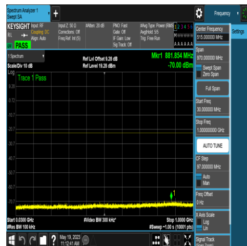
NTNV_N77-3700-3980_PC2_30_100_L_TID18_N S_01_30_1000_#1
