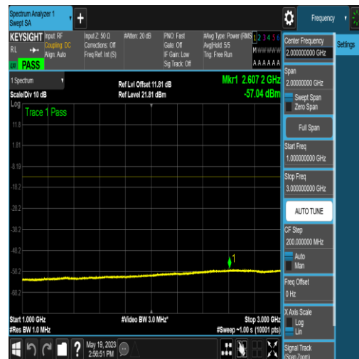
NTNV_N77-3700-3980_PC2_30_15_L_TID16_NS _01_1000_3000_#1
