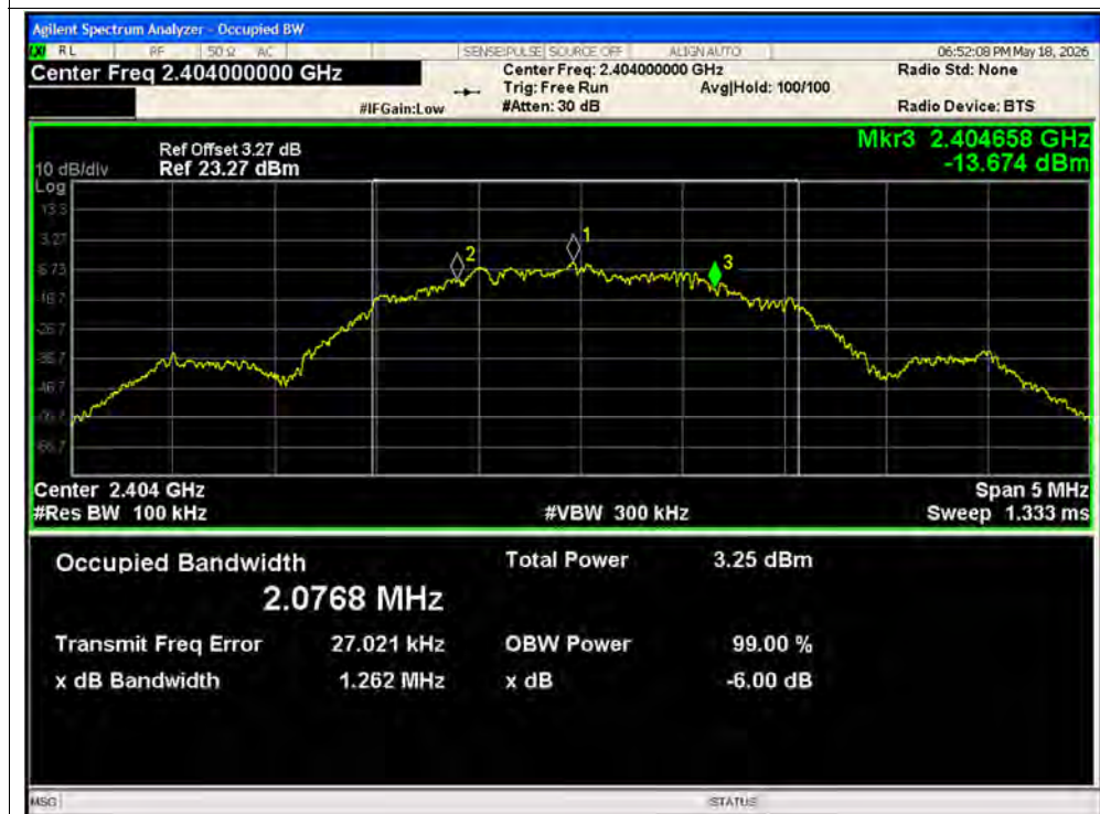
-6dB Bandwidth NVNT BLE 2M 2404MHz Ant1
