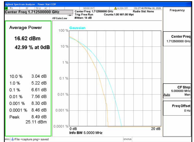
B4 / 5MHz / Low CH / 256QAM
