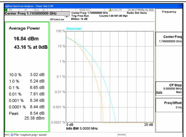
B66 / 5MHz / Mid CH / 256QAM
