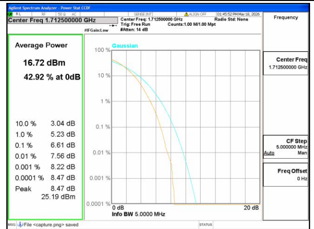
B66 / 5MHz / Low CH / 256QAM
