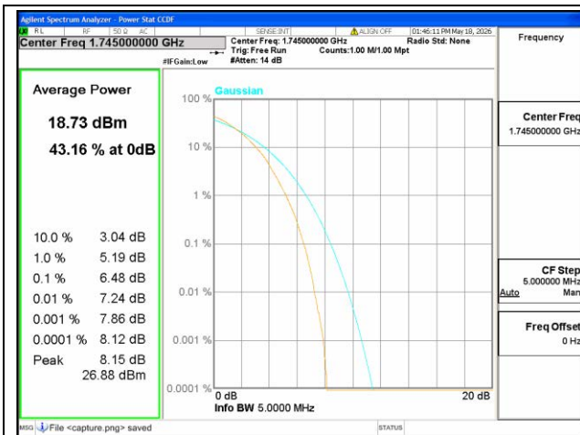
B66 / 5MHz / Mid CH / 64QAM
