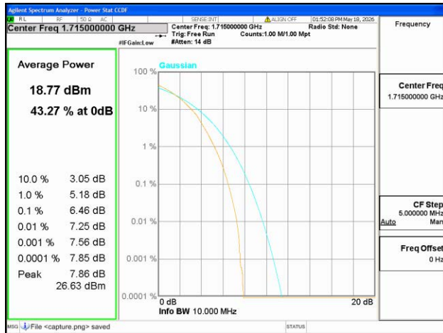
B66 / 10MHz / Low CH / 64QAM
