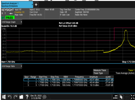
B66 20M 16QAM 1@0 CH 132072
