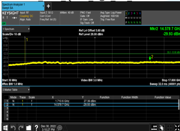
B66 1.4M QPSK 1@0 CH 131979
