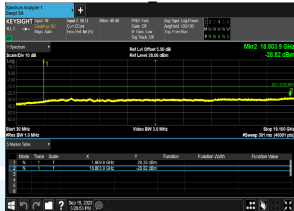
EGPRS1900 Channel810
