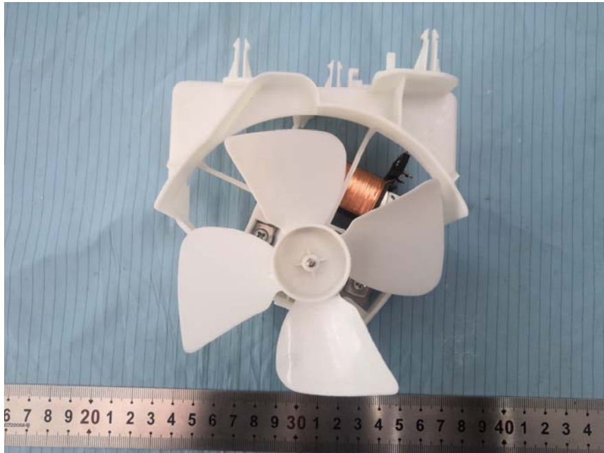
EUT – Fan & Fan Motor Front View
