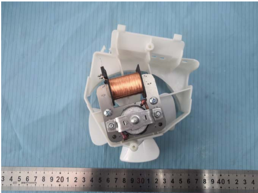
EUT – Fan & Fan Motor Rear View
