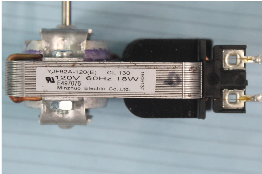
EUT – Fan Motor Label View
