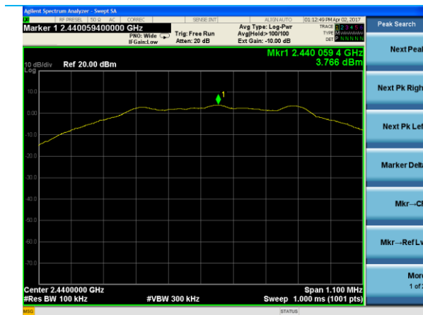
Fundamental
