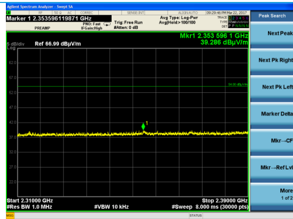
2310-2390 MHz (Average)
