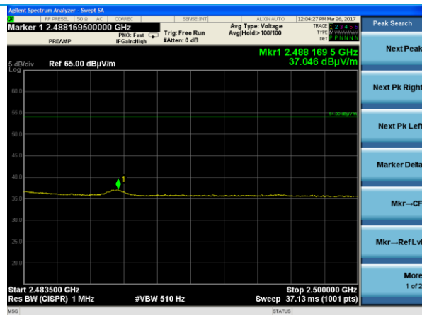
2483.5-2500 MHz (Average)
