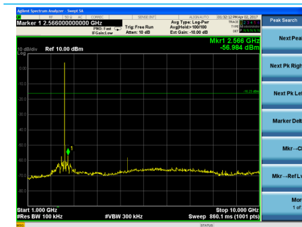
1 GHz - 10 GHz
