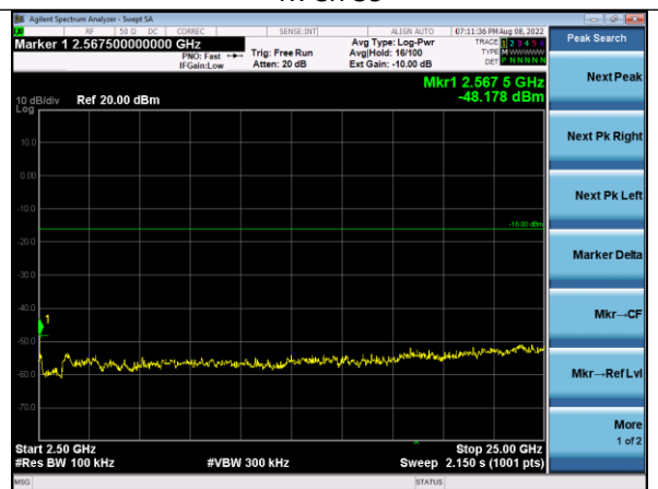
2500-25000 MHz Tx Ch 17
