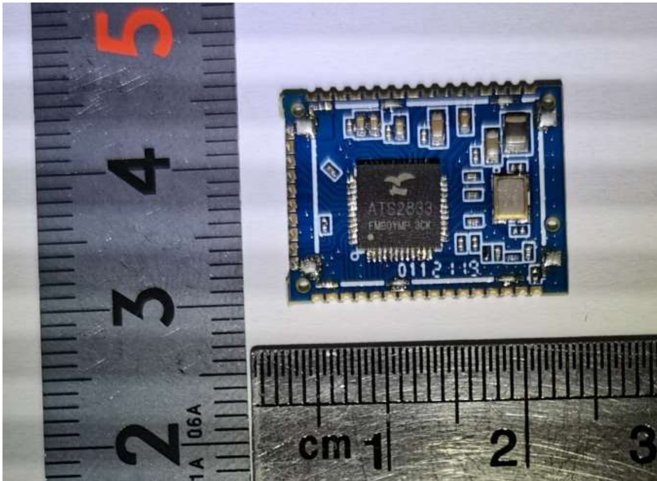
Bluetooth module
