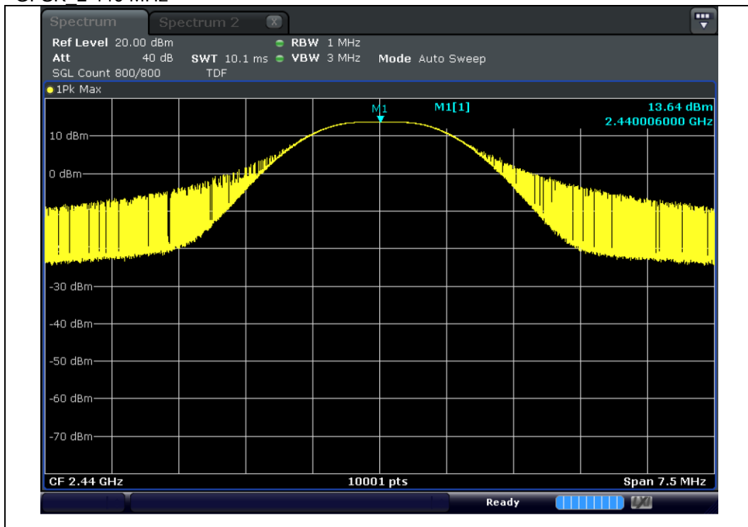
GFSK 2 440 MHz
