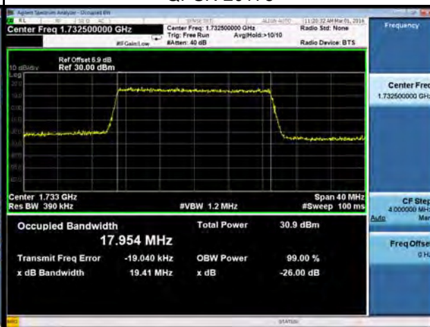
16QAM-20050
