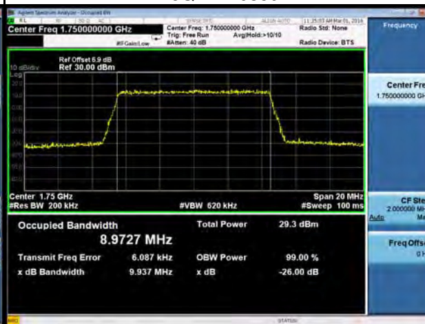
16QAM-20350
