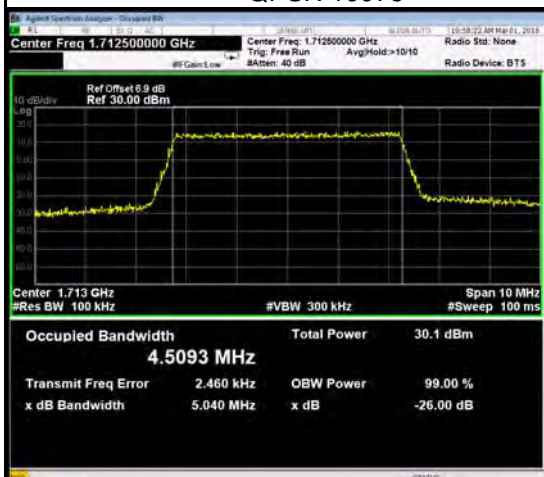
QPSK-20375
