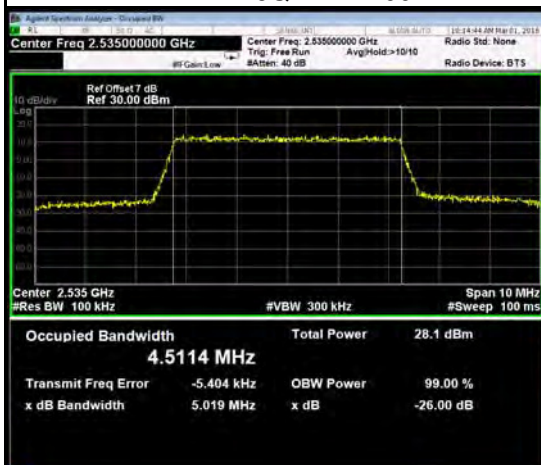
16QAM-21100
