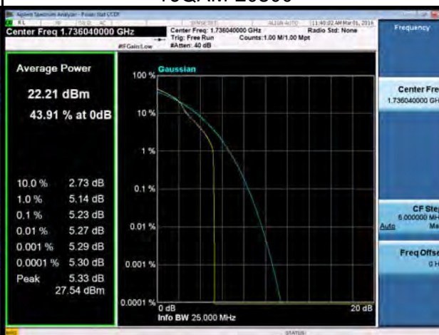
16QAM-20300
