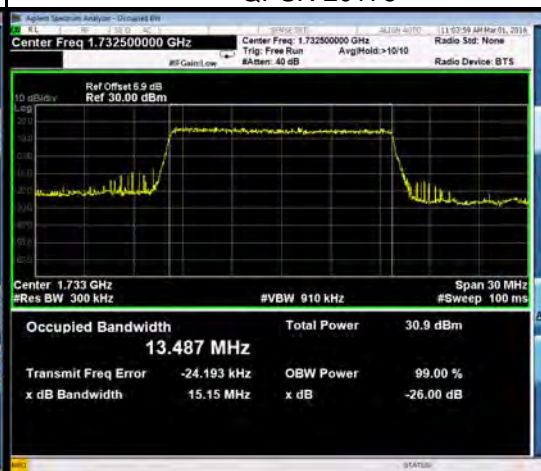
16QAM-20025
