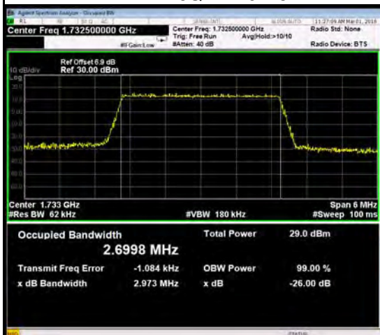
16QAM-20175
