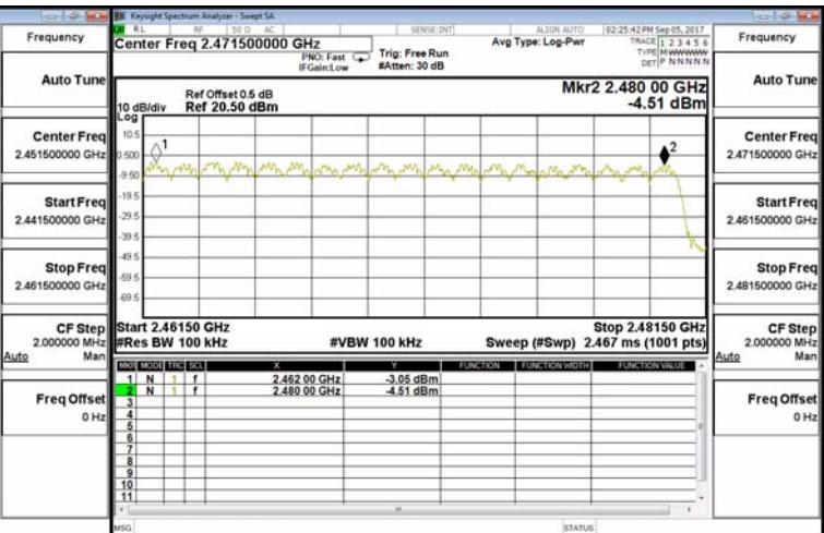
2462-2480MHz
