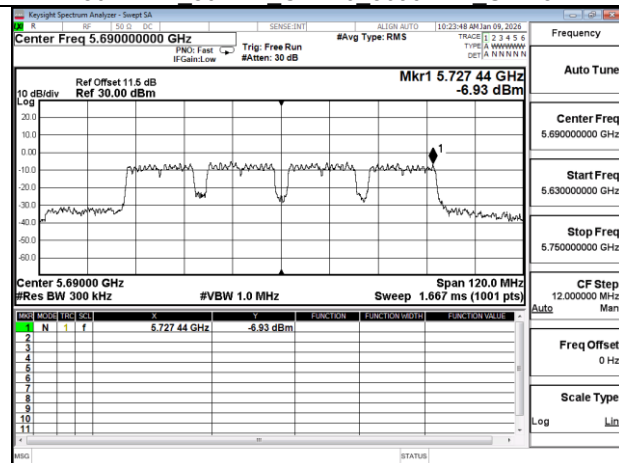
802.11ac 80MHz Chain1 5690MHz UNII 3
