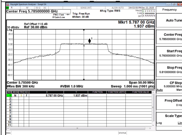
802.11n 20MHz Chain0 5785MHz
