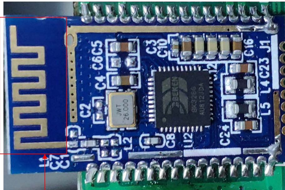
2.4G Antenna
