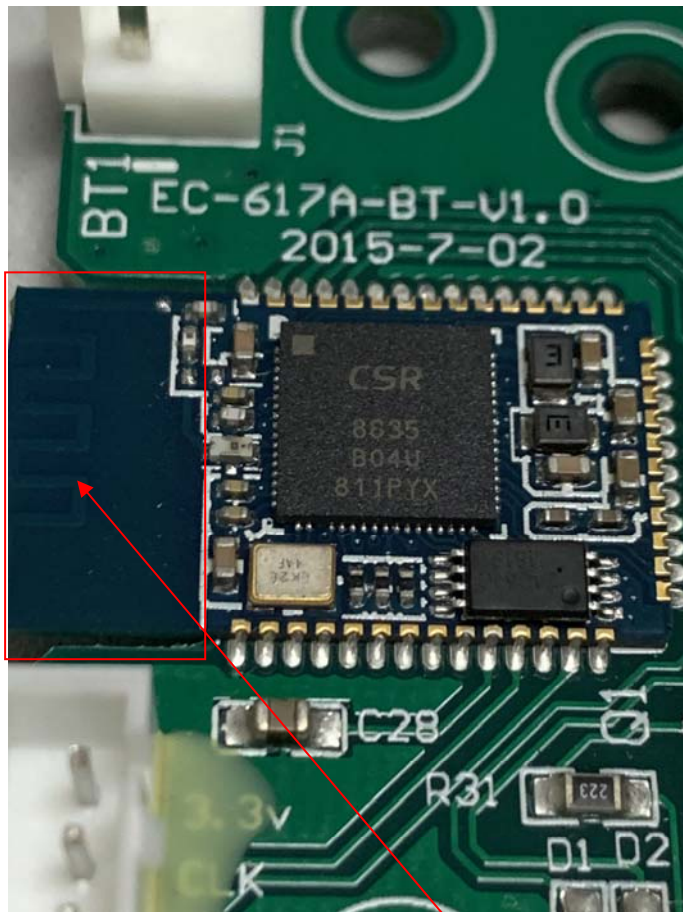
Antenna
