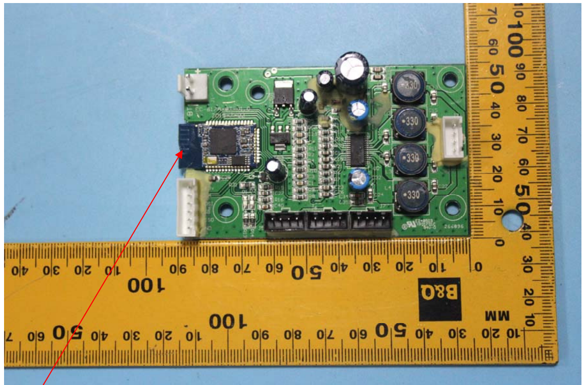
Antenna
