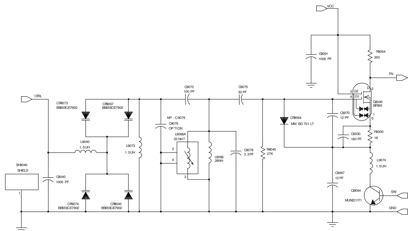
c. VCO 3
