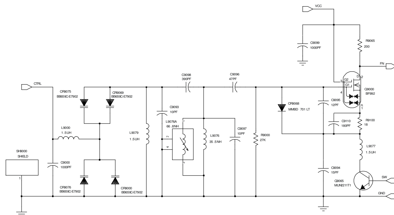
a. VCO 1
