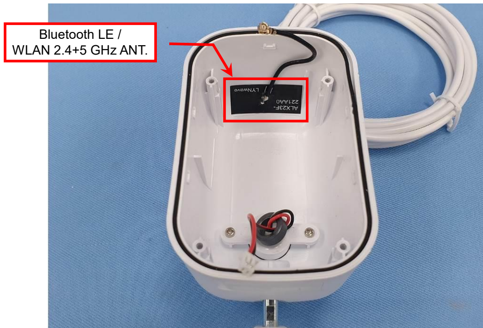
EUT Photo (20)
