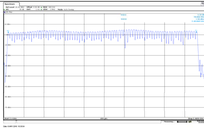
GFSK
