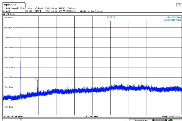
CH01-SE
