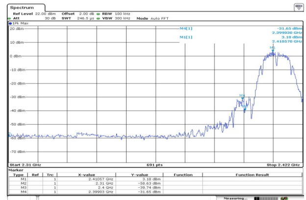
CH01-Bandedge
