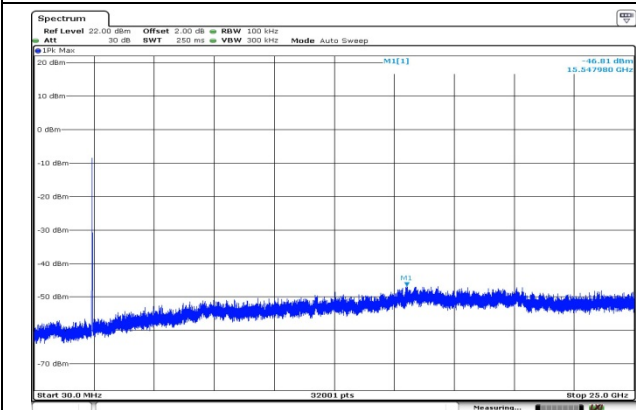
CH06
