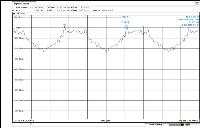
GFSK
