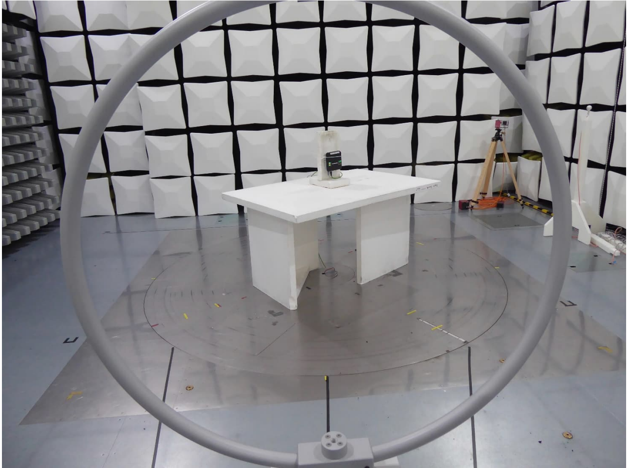
9 kHz – 30 MHz - EUT position 1
