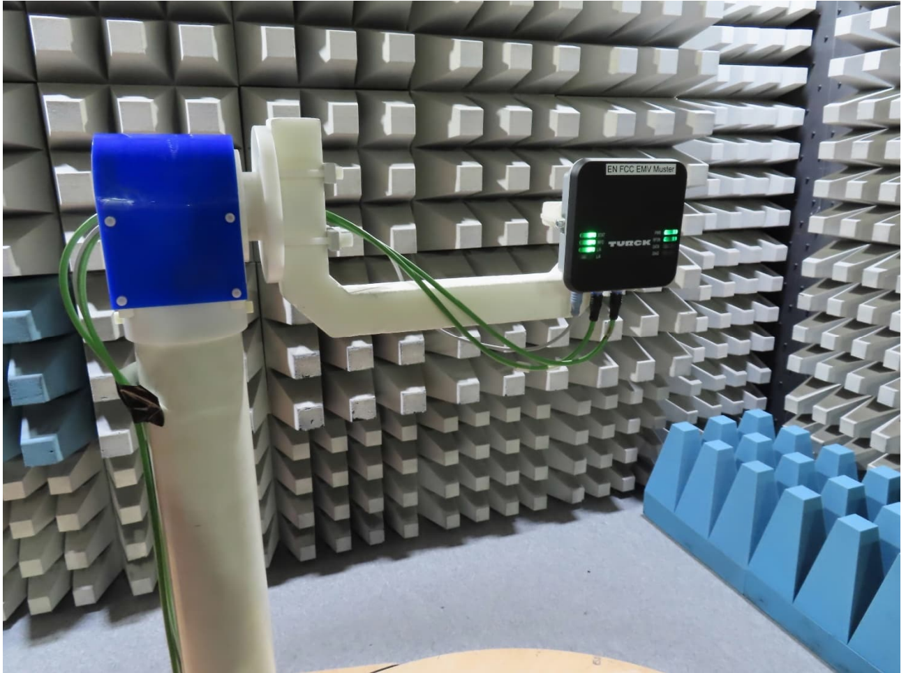
f > 1 \text{ GHz} : EUT setup
