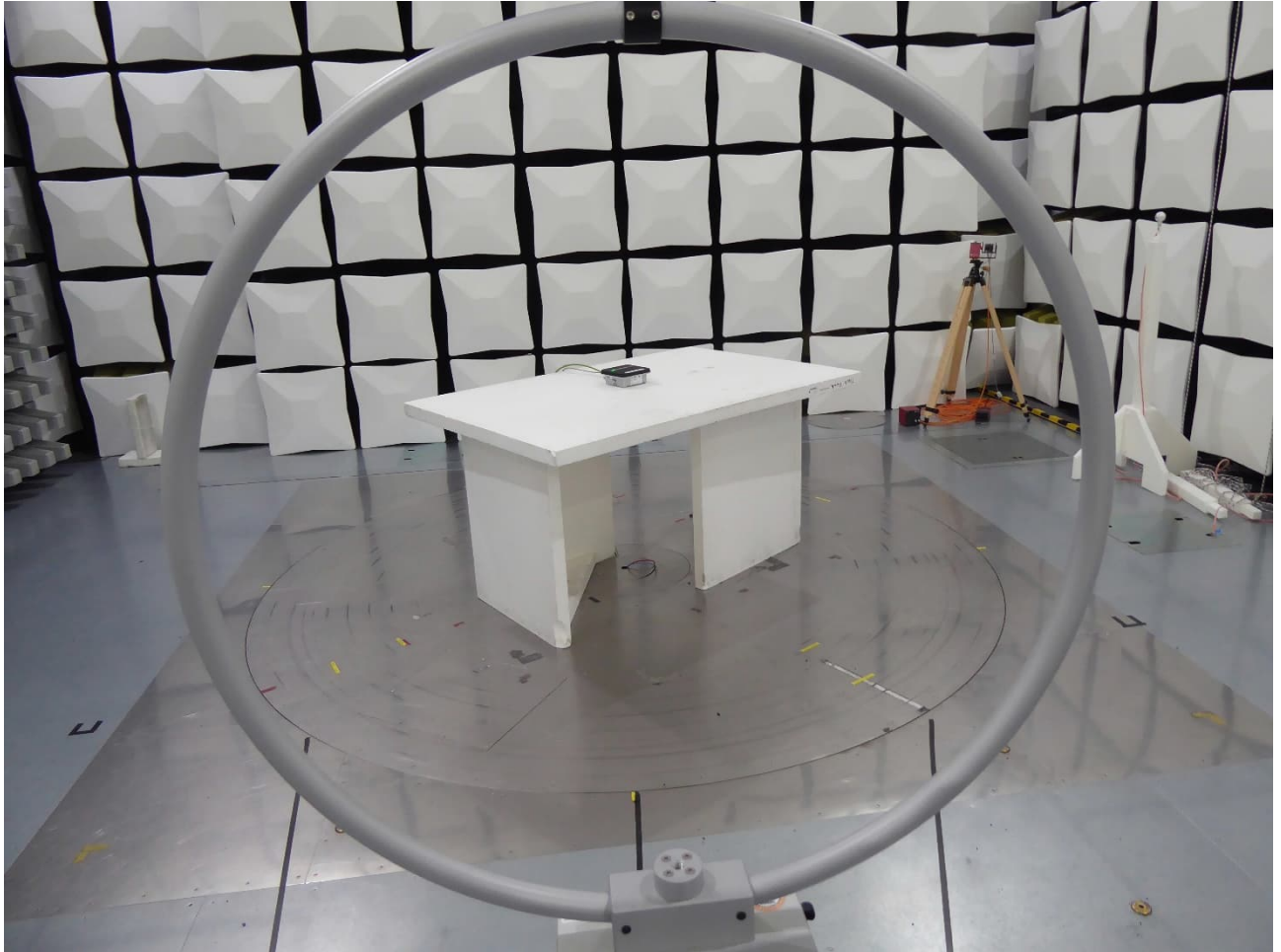
9 kHz – 30 MHz - EUT position 2
