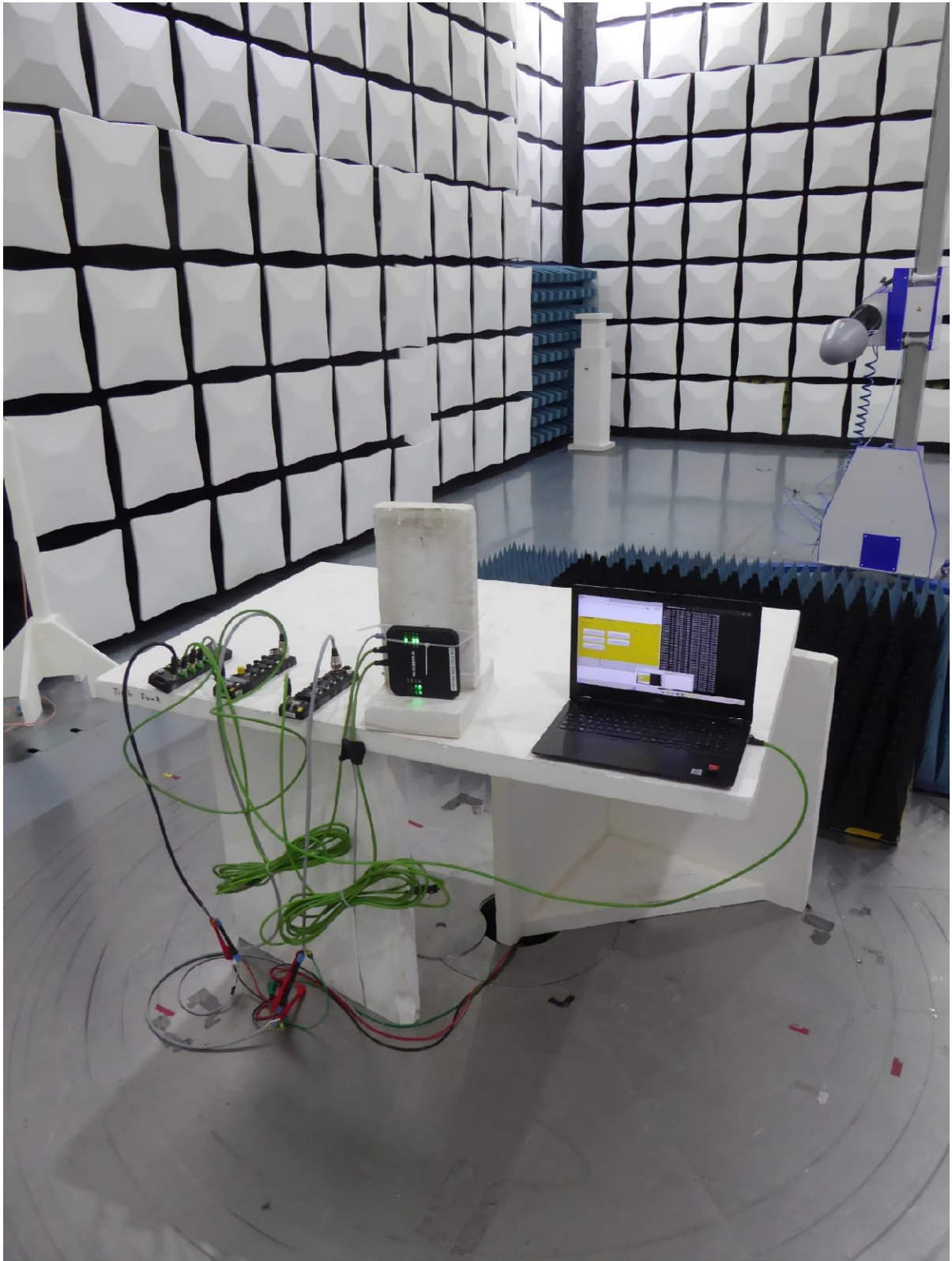
1 GHz - 13 GHz, EUT position 3
