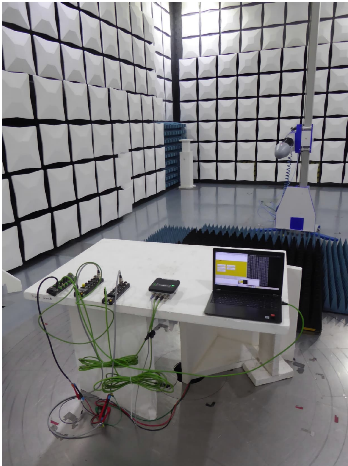
1 GHz - 13 GHz, EUT position 2
