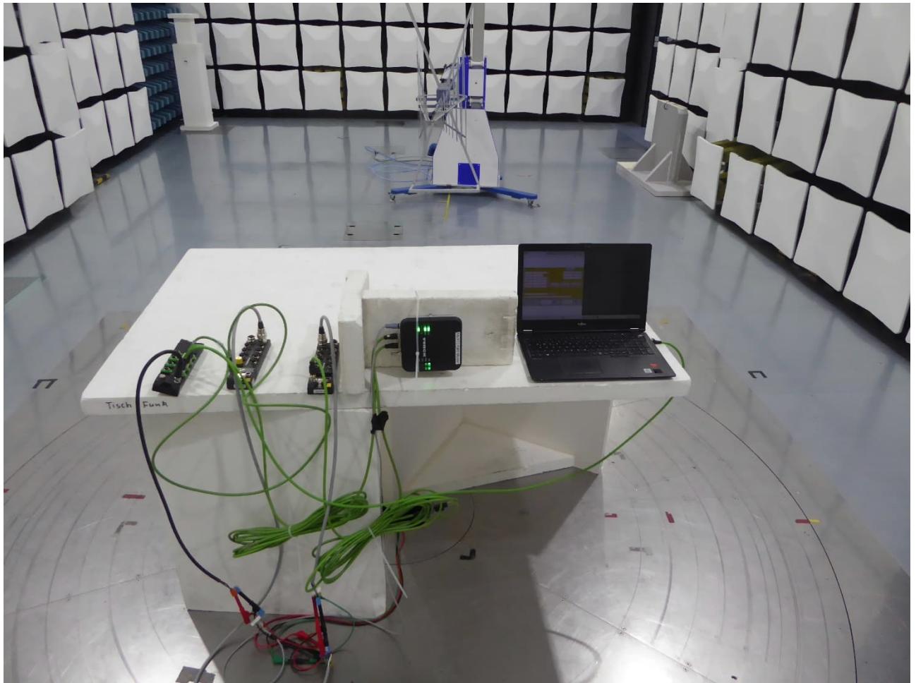
30 MHz - 1 GHz, EUT position 3
