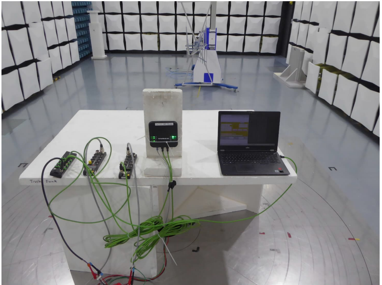
30 MHz - 1 GHz, EUT position 1
