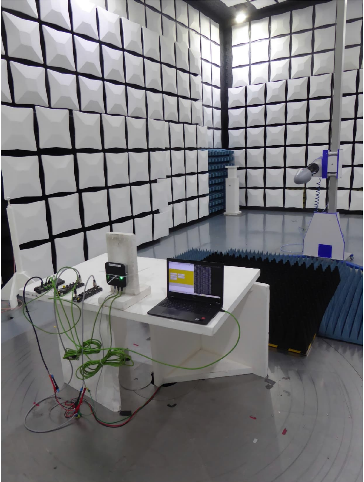
1 GHz - 13 GHz, EUT position 1
