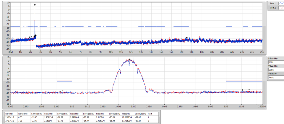
802.11b_Nss1,(1Mbps)_2TX
