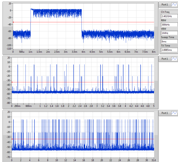
BT-EDR(2Mbps) 2402MHz
