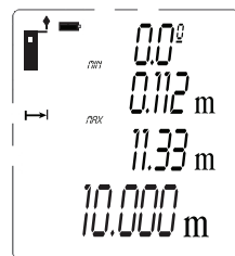
Fig. 6. Resultados del uso de medición continua para alejarse una distancia especificada (10 m) desde una pared
