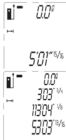
Fig. 5. Tres mediciones directas de distancia en orden de arriba a abajo
