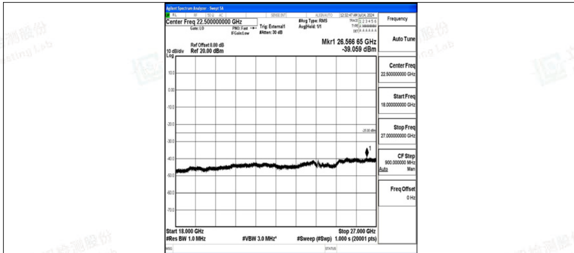
Band38-5MHz-QPSK-38000-25RB#0-18000~27000-PASS
