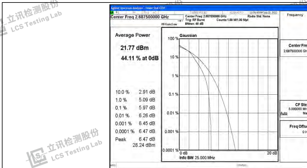
Band41-10MHz-QPSK-39700-50RB#0
