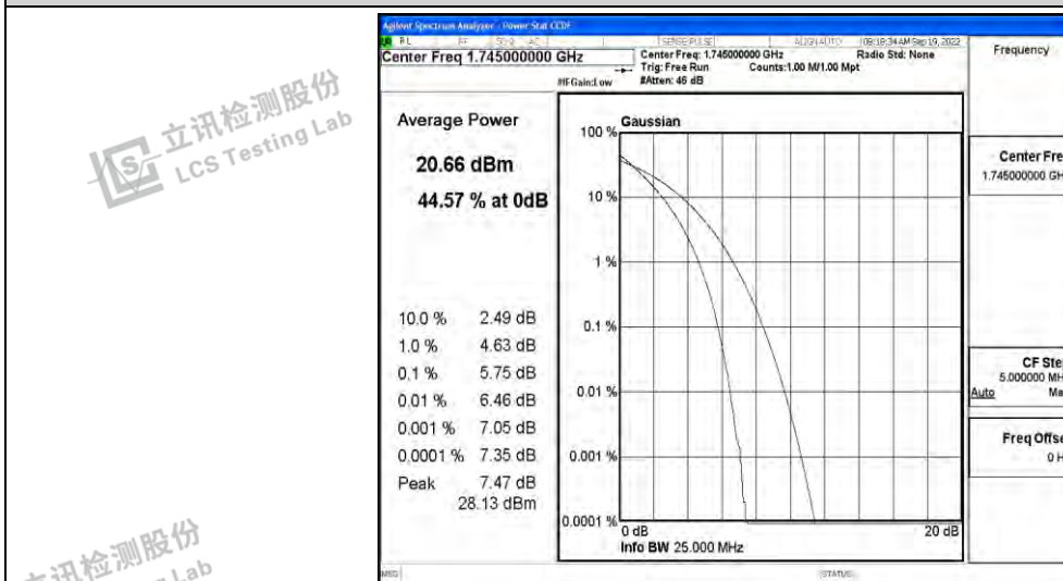
Band66-20MHz-QPSK-132572-100RB#0
