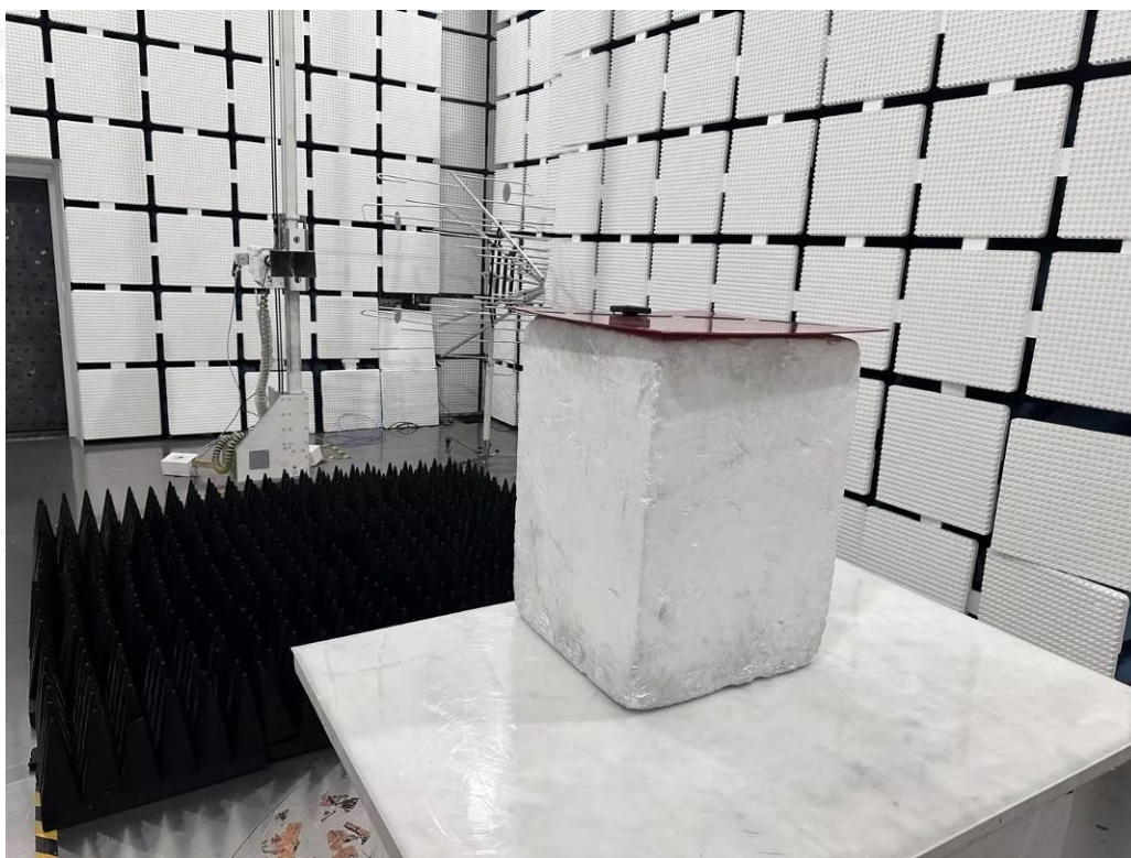
Fig. 3 (Above 1GHz)
