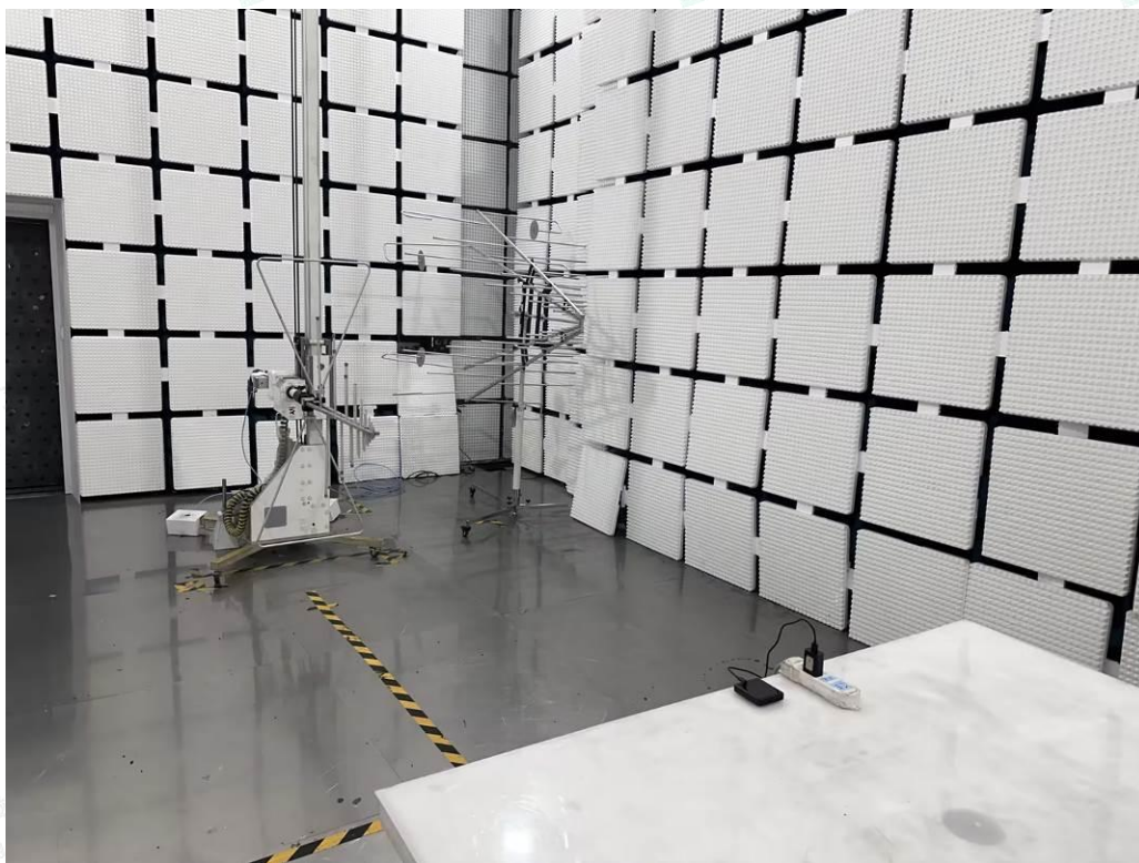
Fig. 2 (30MHz~1GHz)
