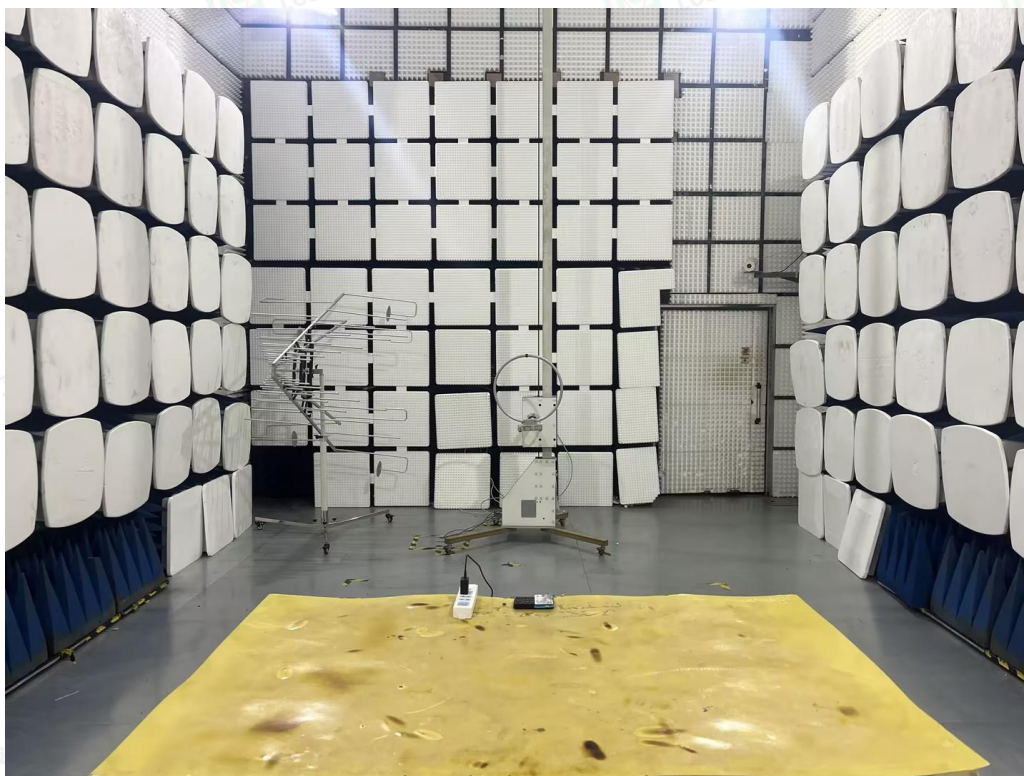
Fig. 1 (Below 30MHz)
