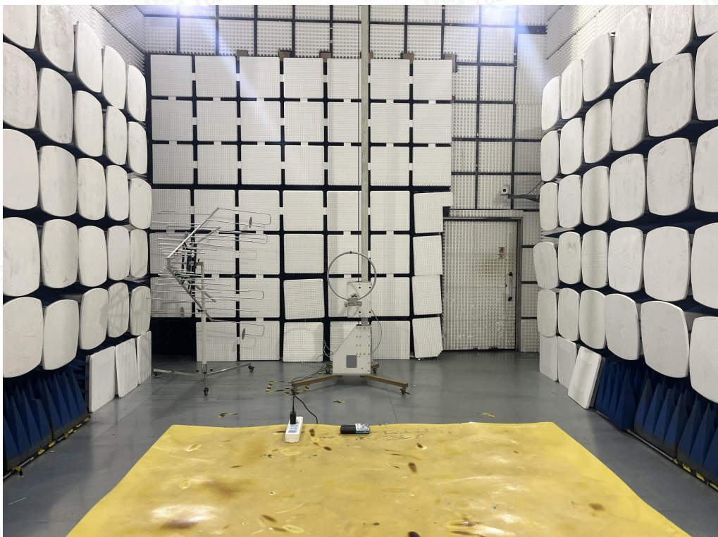
Fig. 1 (Below 30MHz)
