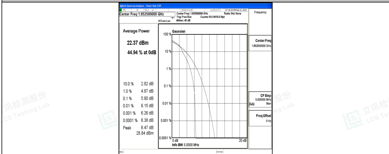
Band2-5MHz-16QAM-18625-1RB#0-PASS
