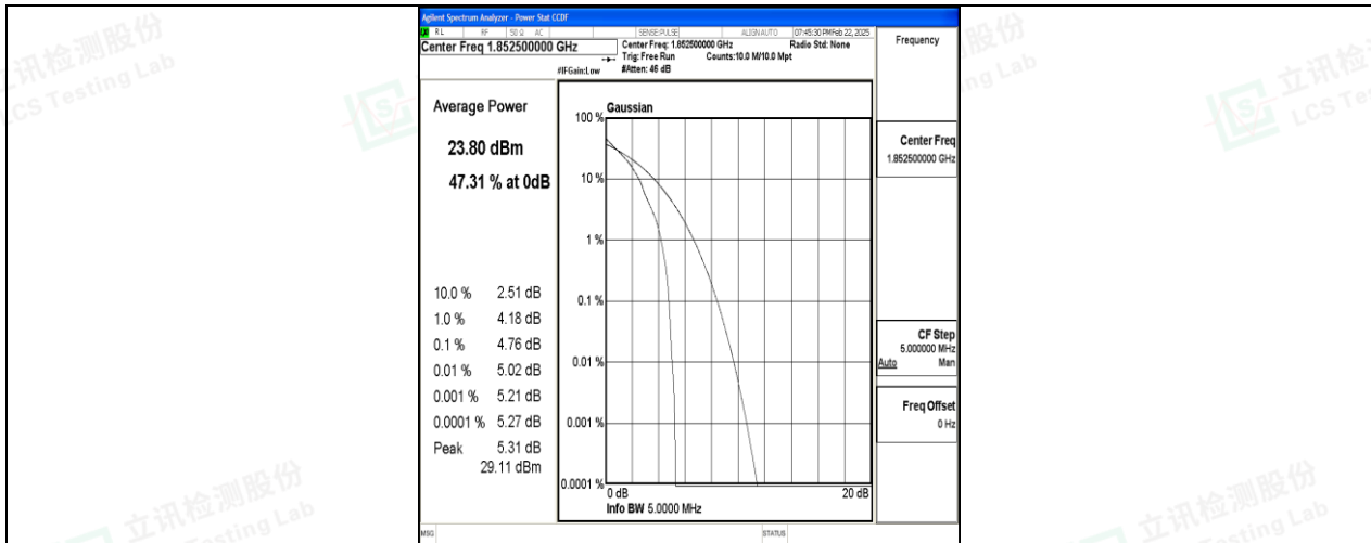
Band2-5MHz-QPSK-18625-1RB#0-PASS
