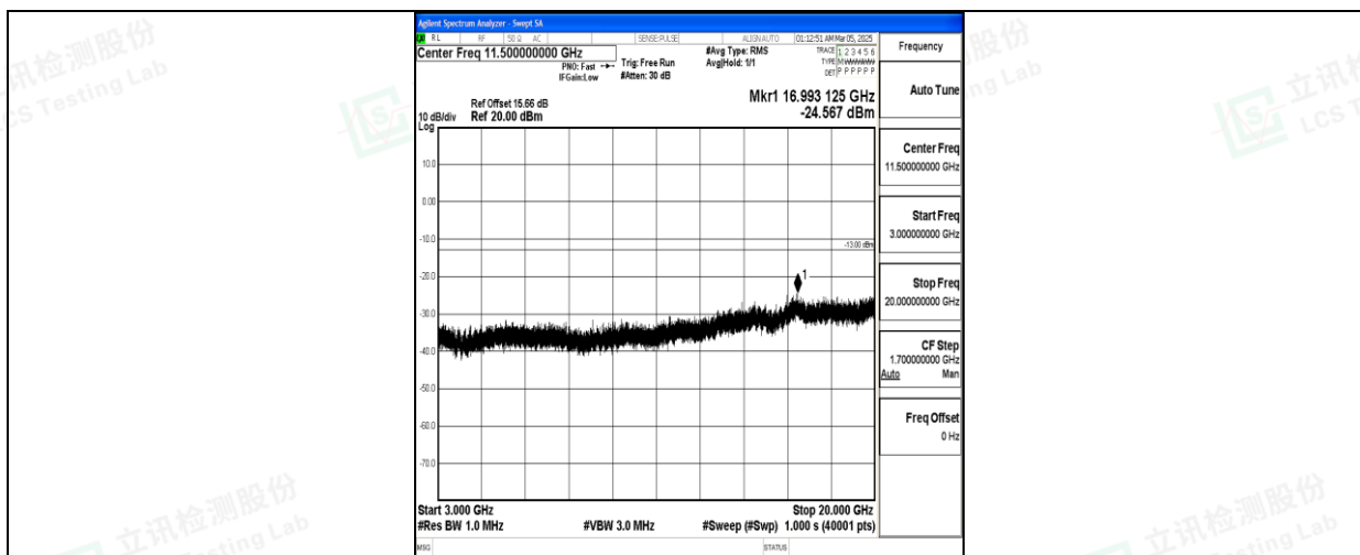
Band66 15MHz QPSK 132047 1RB#0 3000~20000 3000~20000
