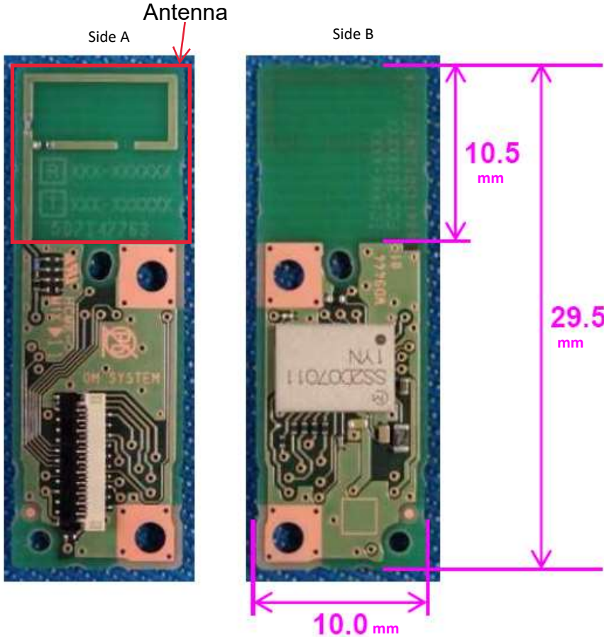
S0123WIFI-PCA External View
