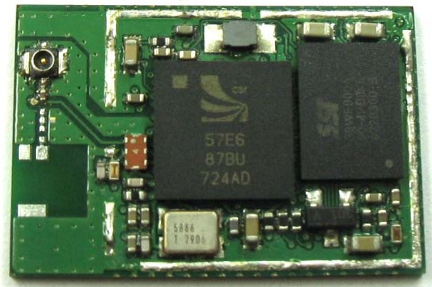
WT32-A
