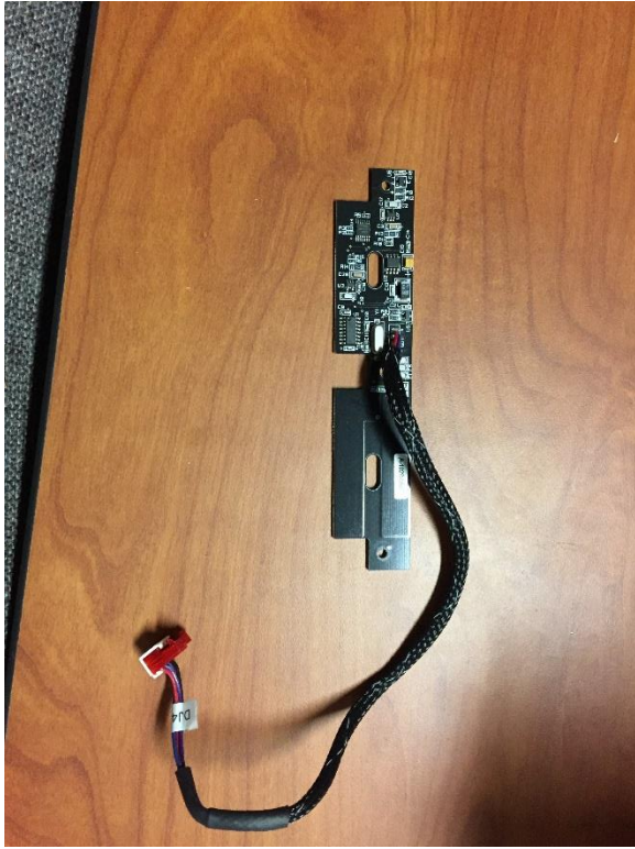
RFID Board – Actual EUT
