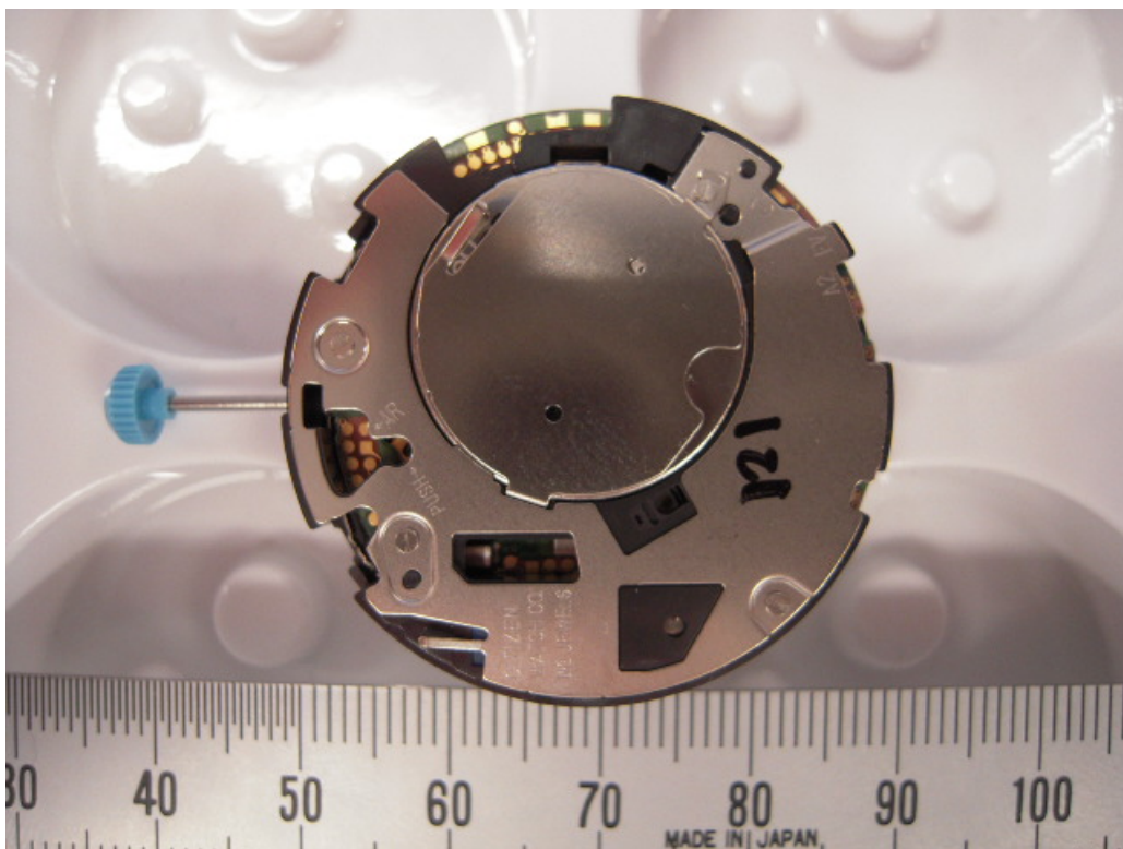
Bottom
