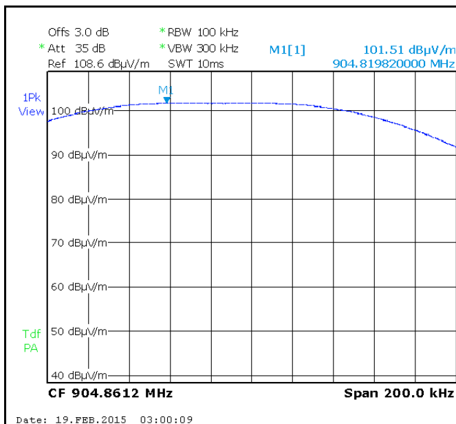
PSD - Low CH
