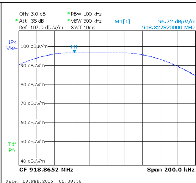
PSD - Mid CH
