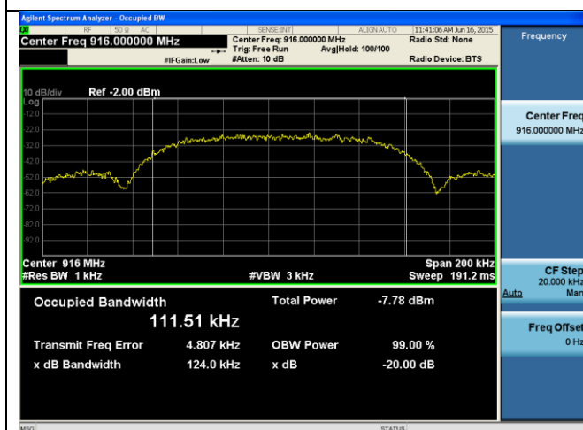
20dB BW -916.00MHz-100kbps
