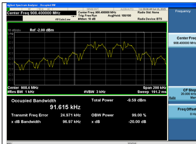
20dB BW -908.40MHz-9.6kbps
