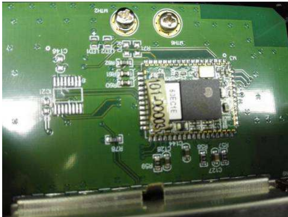
BT module
