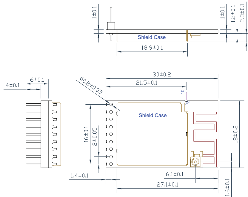
Fig. 2-6 Dimensions
