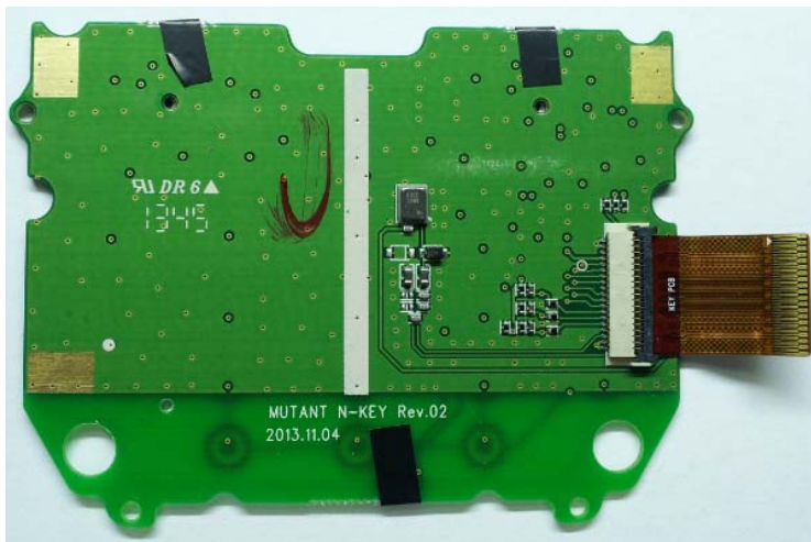
10. Numeric Key PCB (SKU1 : NX4-1DGN-0-E / SKU5 : NX4-2DGN-0-E)
