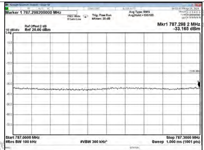
Upper 700 Band UL-LTE Right Side AGC+10dB
