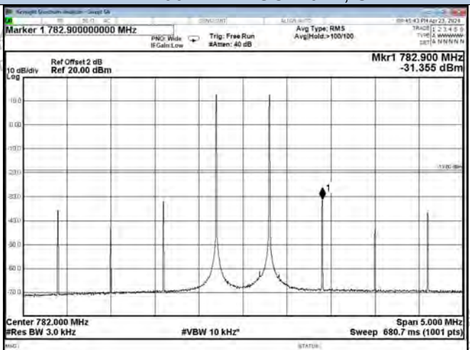
Upper 700 Band AGC+10dB, UL
