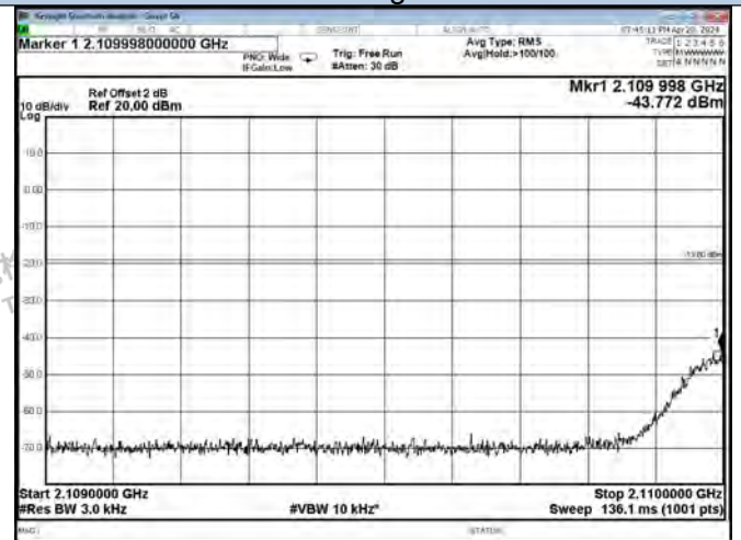
AWS Band DL-GSM Left Side AGC+10dB
